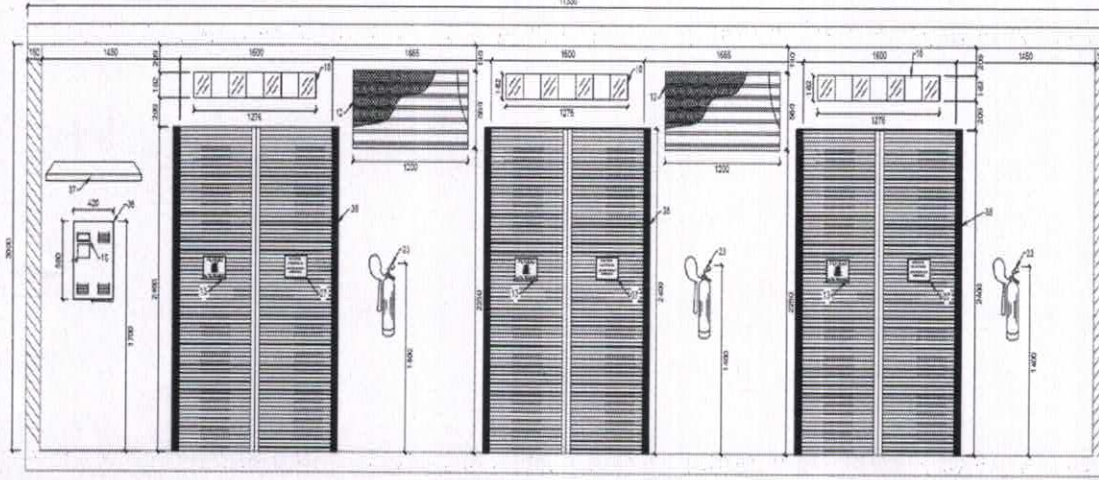
VISTA FRONTAL SALA - TRANSFORMADORES 01 E 02 - ESCALA 1:25 - COTAS: mm
